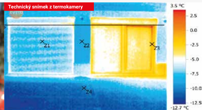
Technický snímek z termokamery
